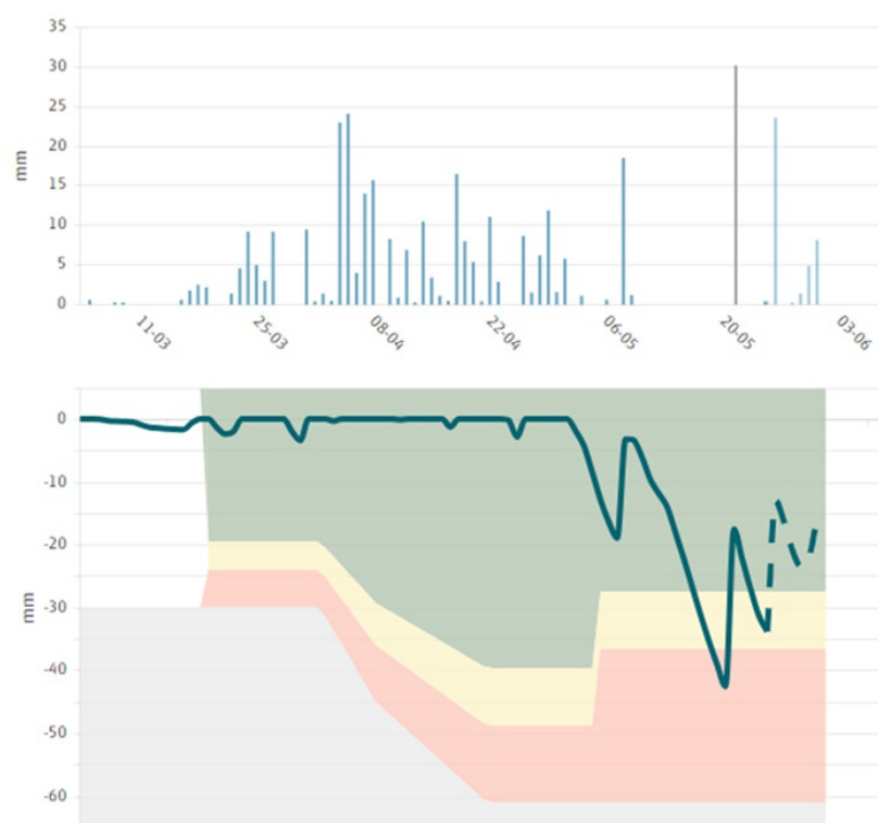
Figur 2 Vandbalance i vinterhvede.
